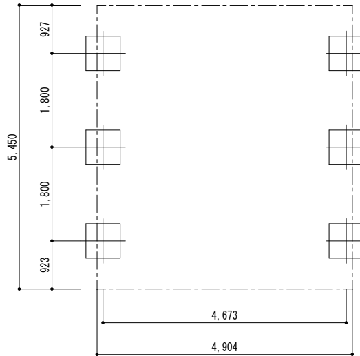
■ 基礎配置図
